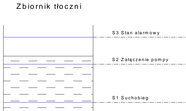
Rys.1. Rysunek obrazujący pracę przepompowni
