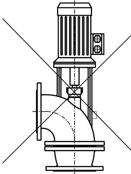
Rys.1 Przykład niewłaściwego zainstalowania agregatu
